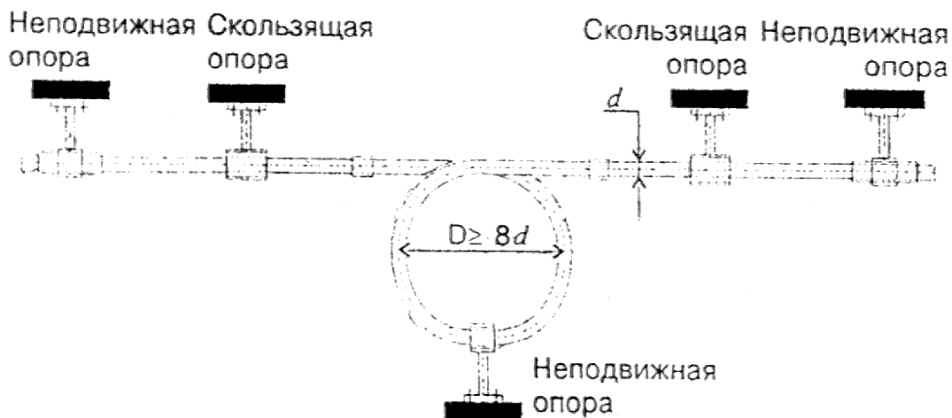
Рис. 2.6. Петлеобразный компенсатор
