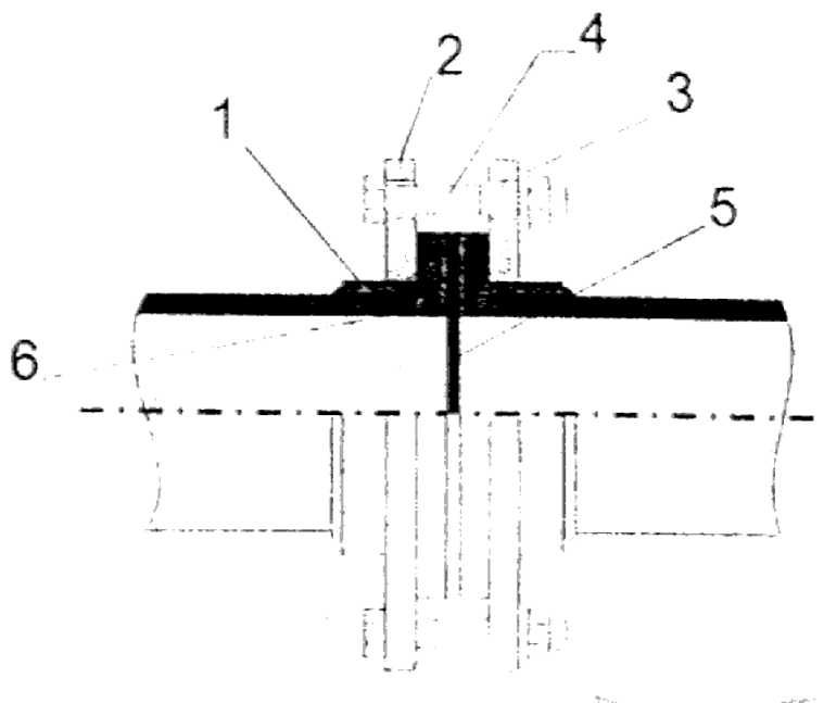
Рис. 5.3. Соединение труб из PPRC на свободных фланцах
