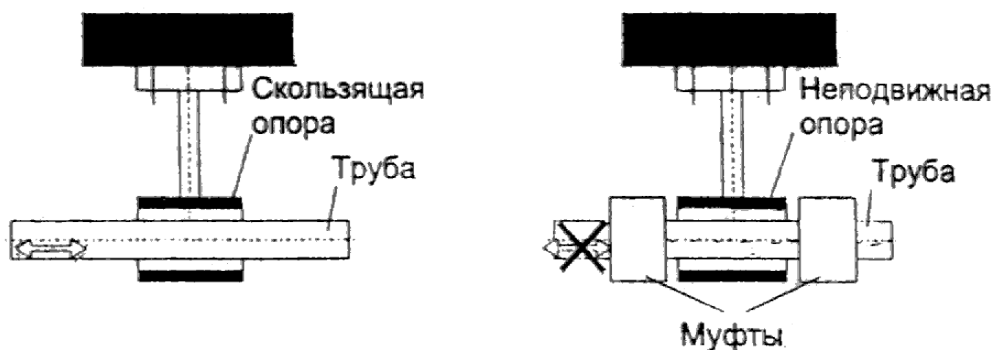
Рис. 4.1. Виды опор
